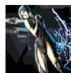
Uranus
